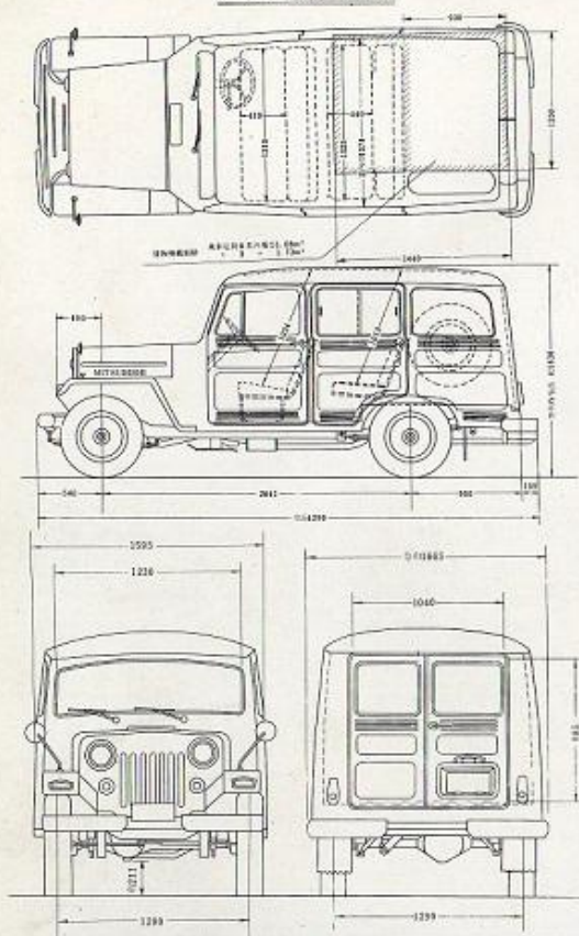
J 30 外観三视图
